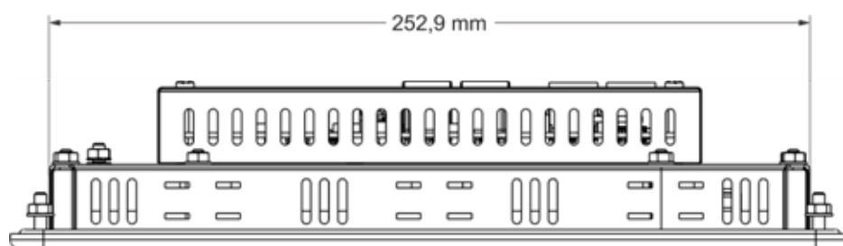
Maßblatt B-Primis DC-Pro 10
