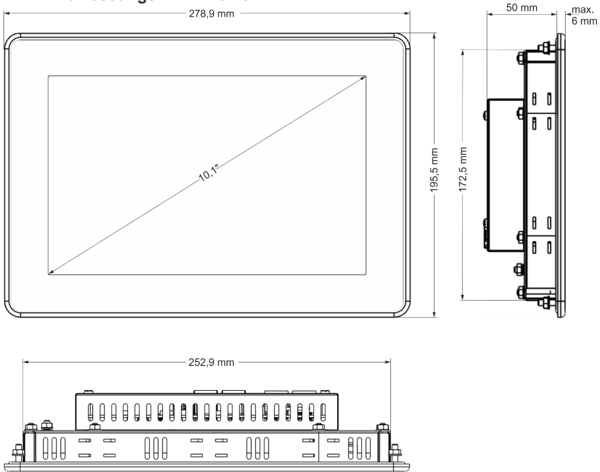
Abb. 11: Abmessungen DC-Pro 10
