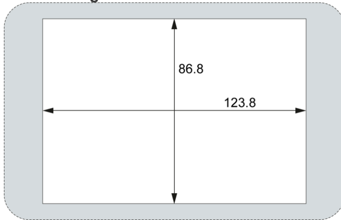
Abb. 6: Montageausschnitt DC-Pro 4
