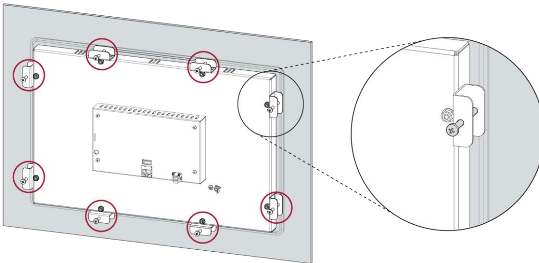
Abb. 24: Spannklammern festschrauben
