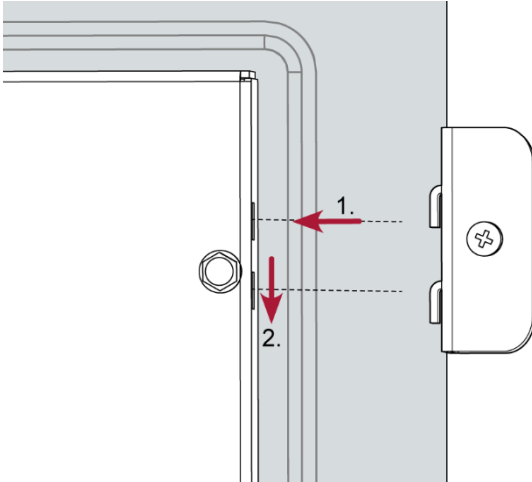
Abb. 23: Spannklammer einhängen (Rückseite)
