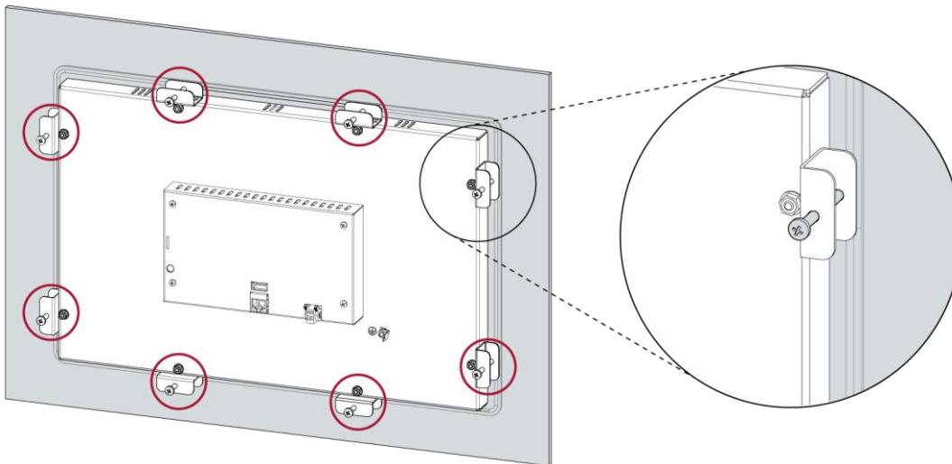
Abb. 21: Spannkammern festschrauben
