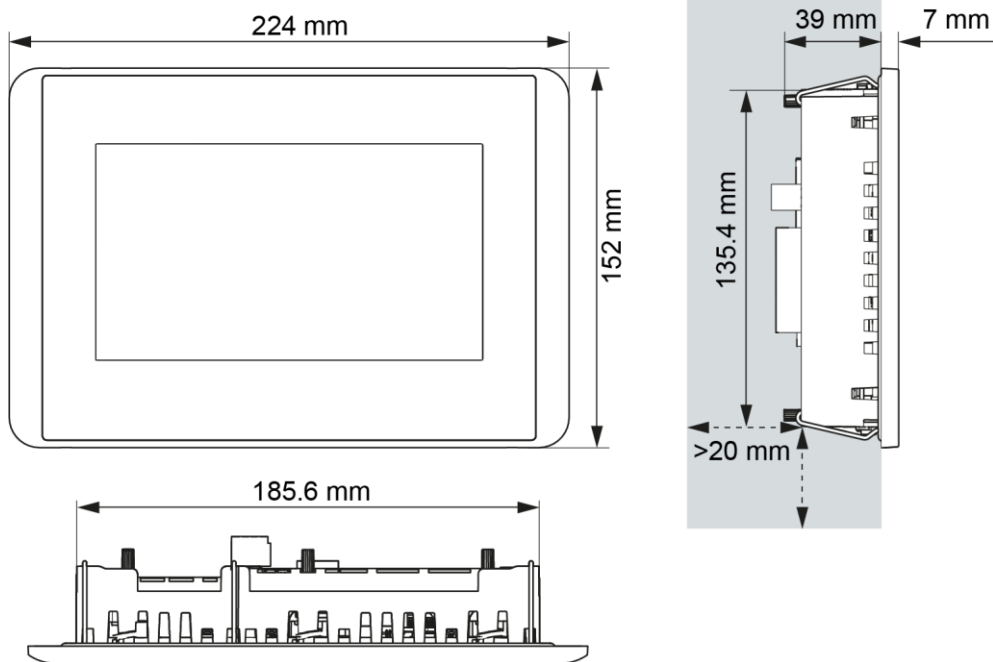
Abb. 7: Abmessungen DC-Pro 7
