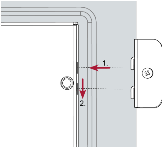
Abb. 20: Spannkammern einhängen (Rückseite)
