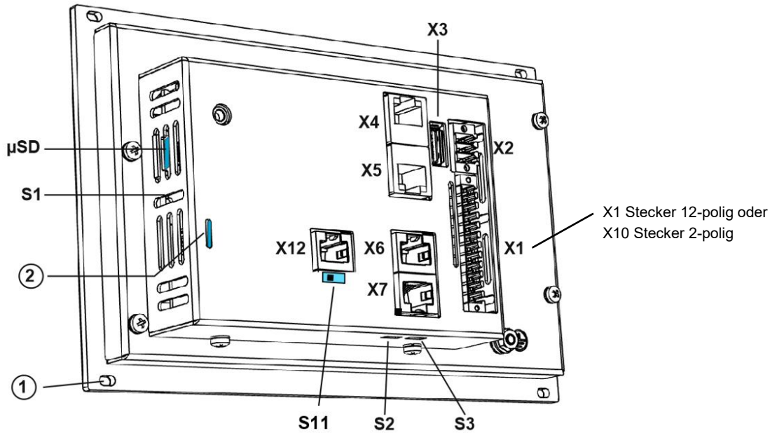
Abb. 3: Übersicht DC-Rack 7 (Rückseite)
