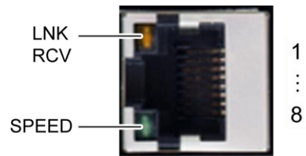
Abb. 39: Ethernet Schnittstelle X4
