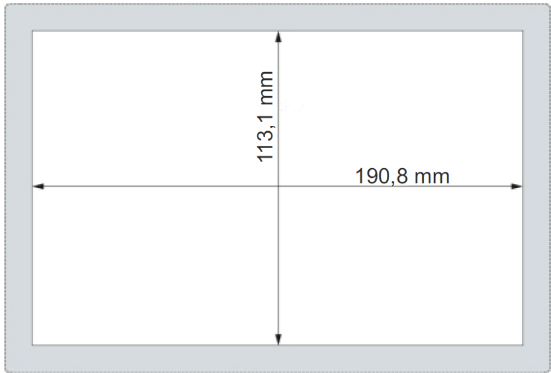
Abb. 10: Montageausschnitt DC-Rack 7
