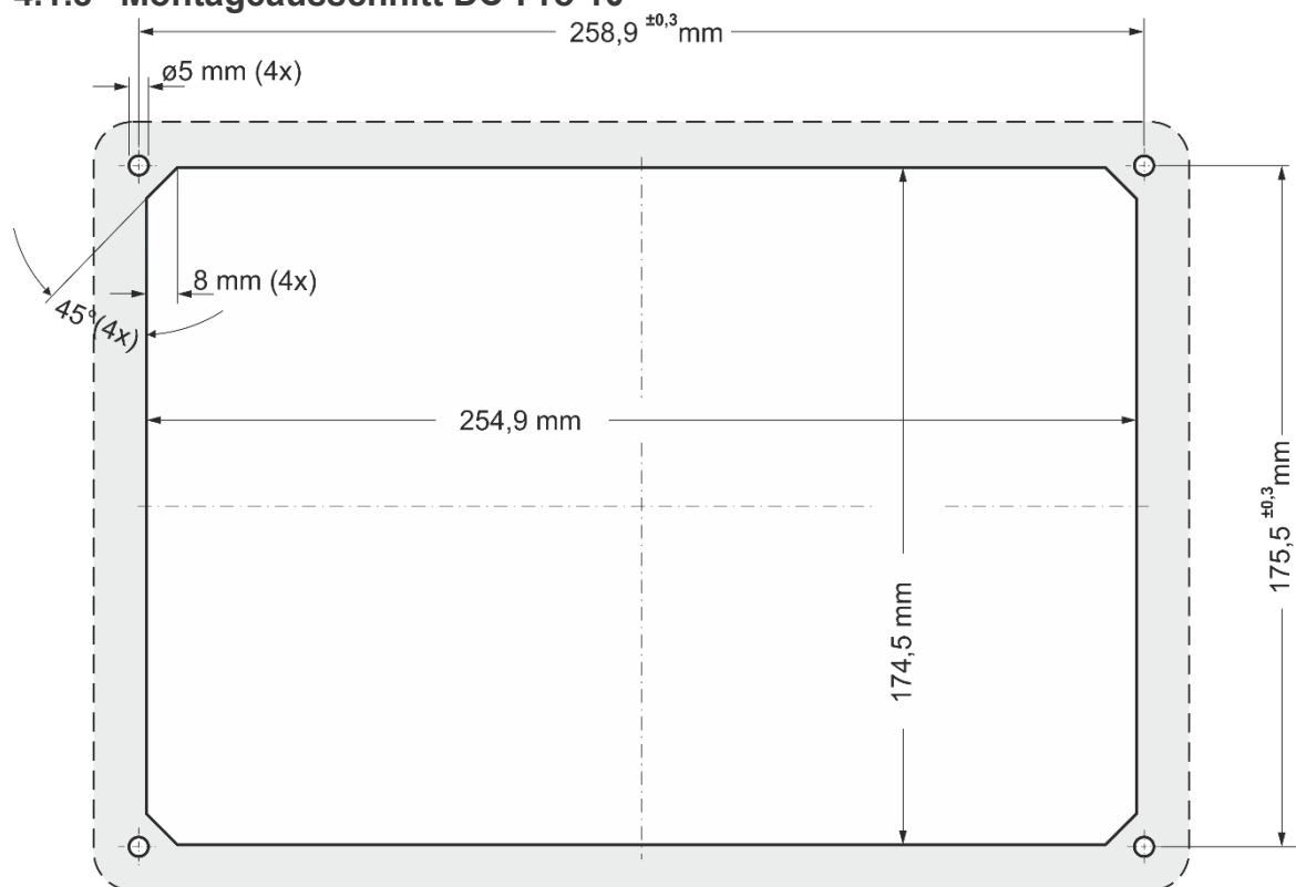
Abb. 12: Montageausschnitt DC-Pro 10
