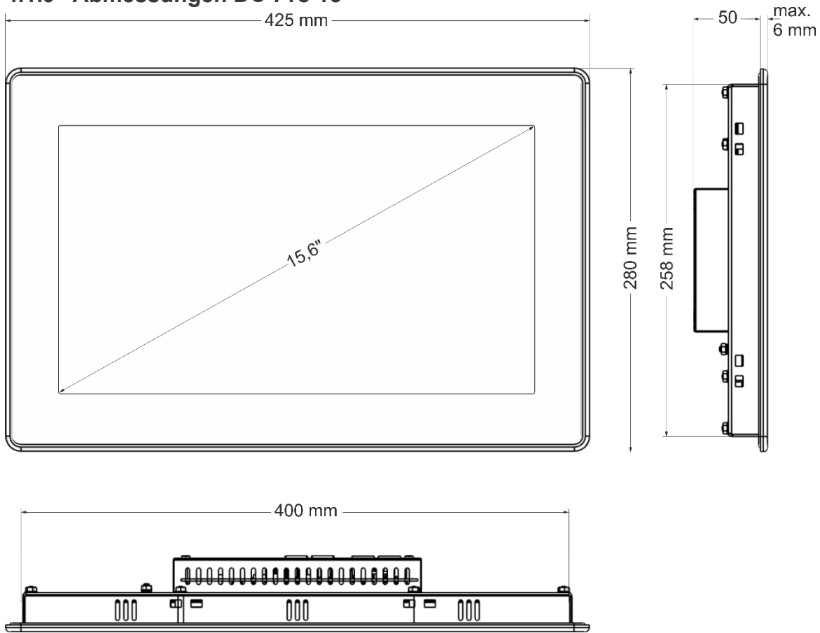
Abb. 13: Abmessungen DC-Pro 15
