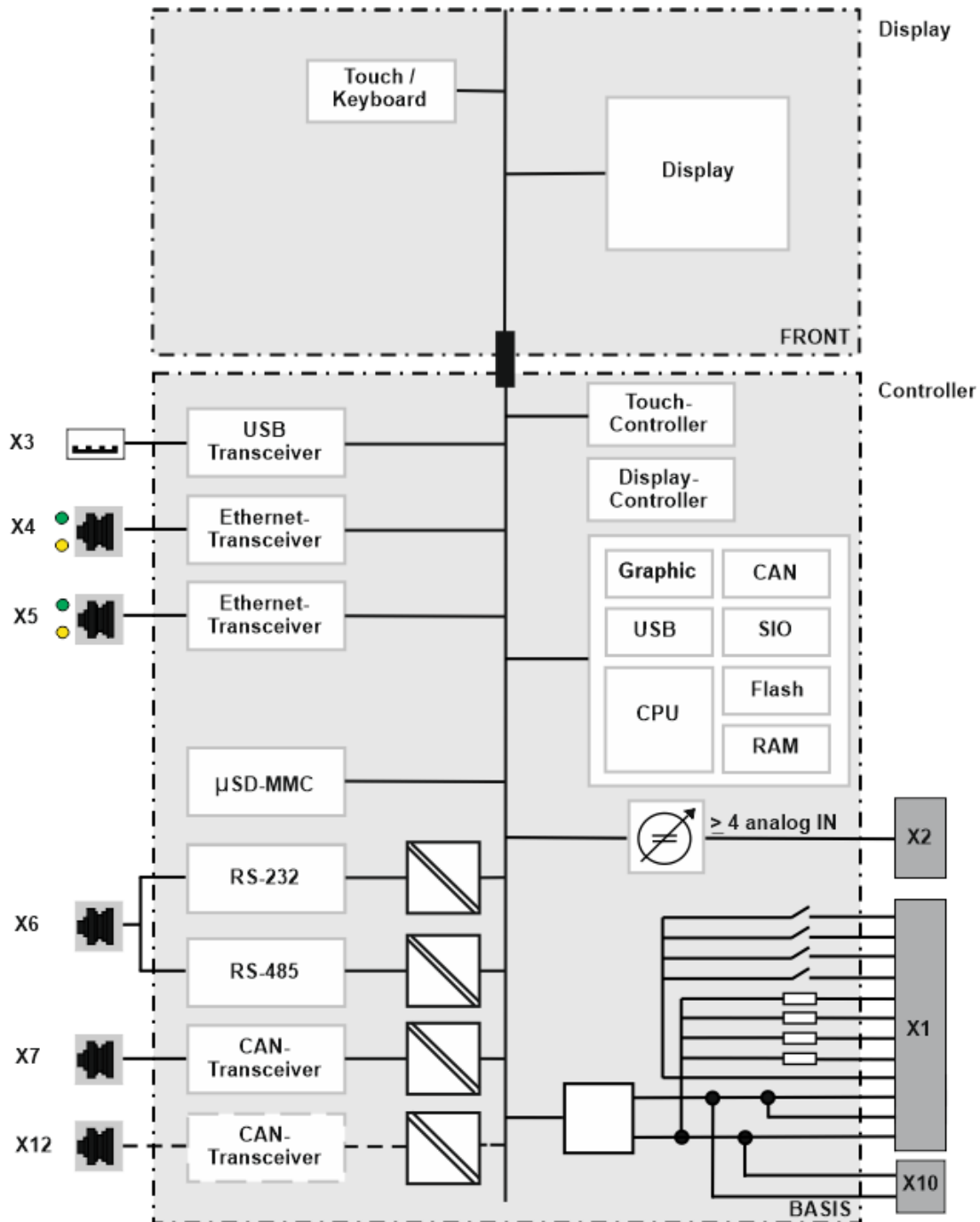
Abb. 28: Blockschaltbild DC-Pro
