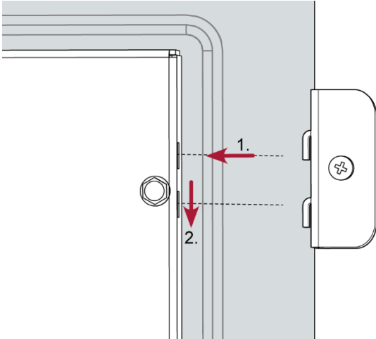
Abb. 23: Spannklammer einhängen (Rückseite)
