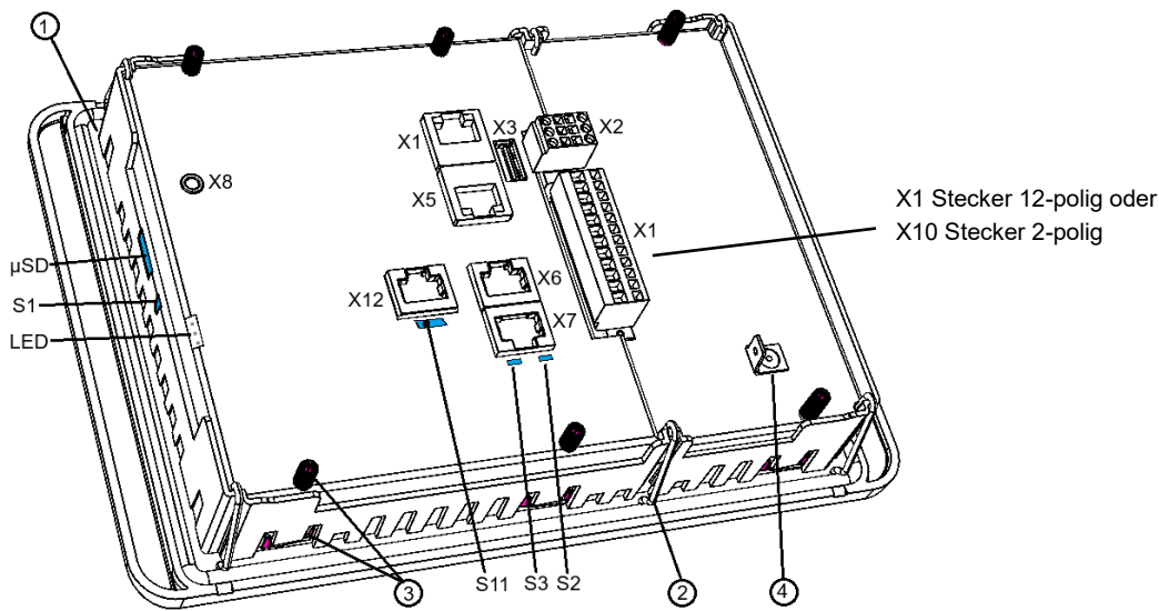
Abb. 2: Übersicht DC-Pro 7 (Rückseite)
