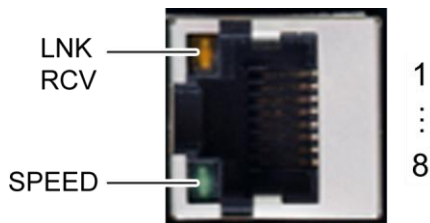
Abb. 40: EtherCAT-Schnittstelle X5
