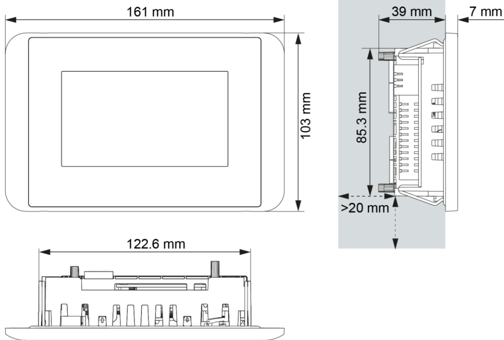
Abb. 5: Abmessungen DC-Pro 4
