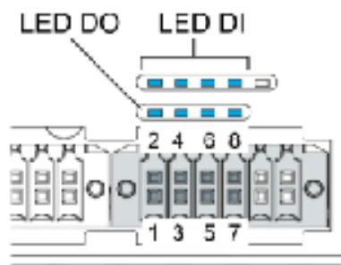
Abb. 30: Digitale Ein- und Ausgänge DC-Pro Stecker X1 mit LEDs 1 bis 8, zweireihig
