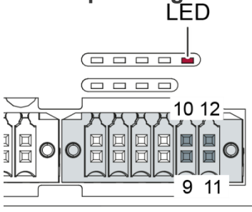
Abb. 27: Spannungsversorgung DC-Pro 10/15 Stecker X1 mit Power-LED
