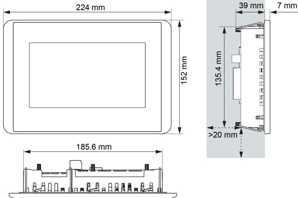
Abb. 7: Abmessungen DC-Pro 7
