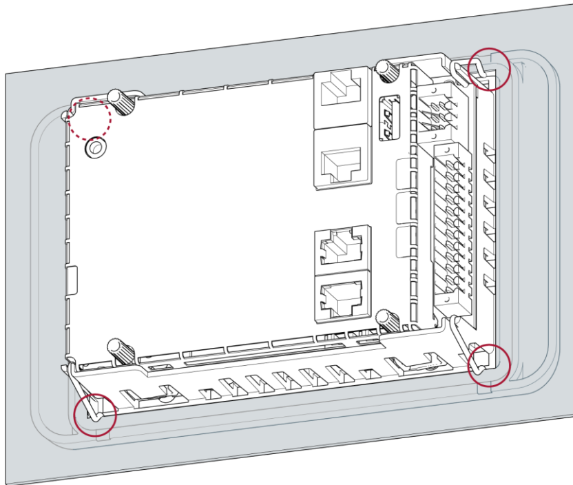
Abb. 17: Gerät im Montageausschnitt eingerastet, Beispiel mit 2 Spannbügel
