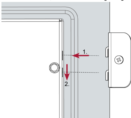
Abb. 20: Spannkammern einhängen (Rückseite)
