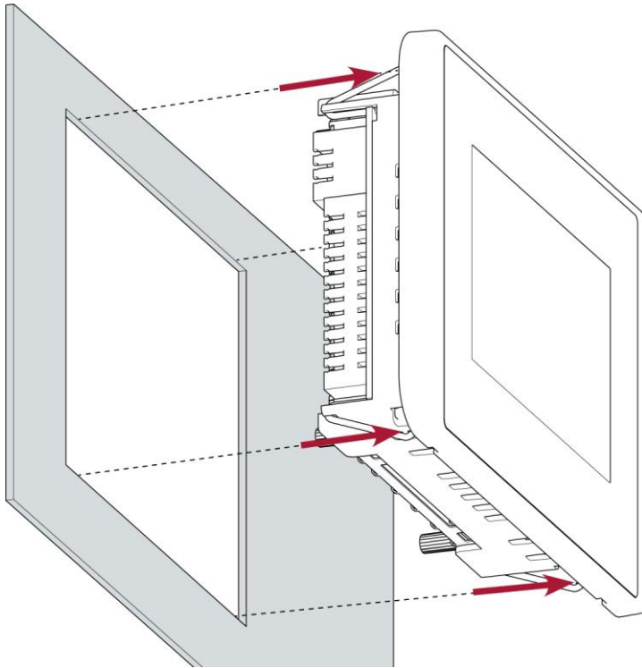
Abb. 54: Gerät aus Montageausschnitt schieben
