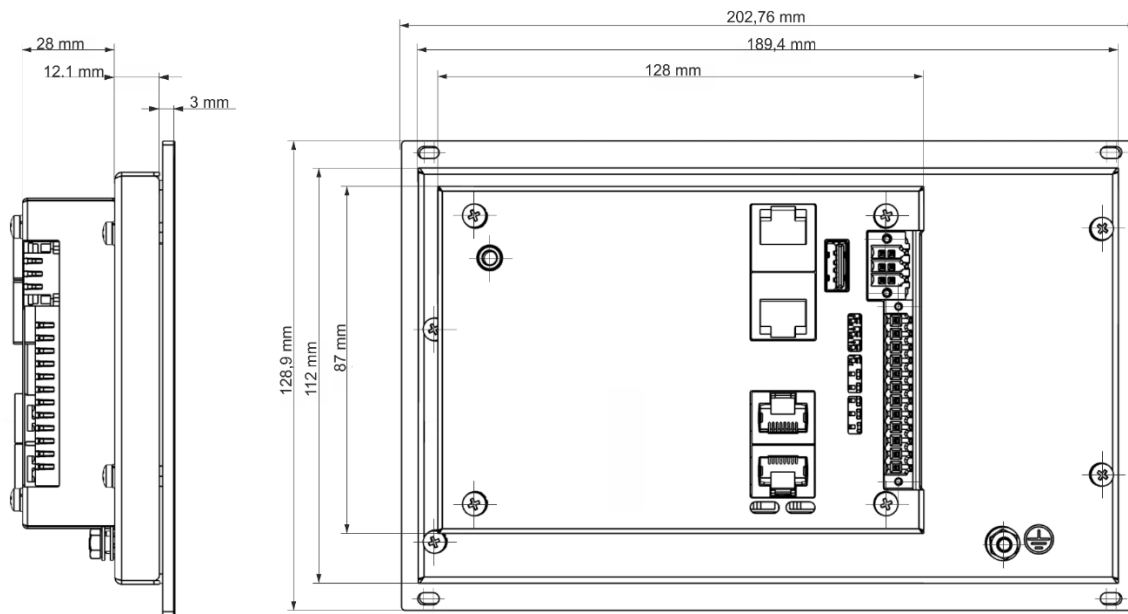
Abb. 9: Abmessungen DC-Rack 7
