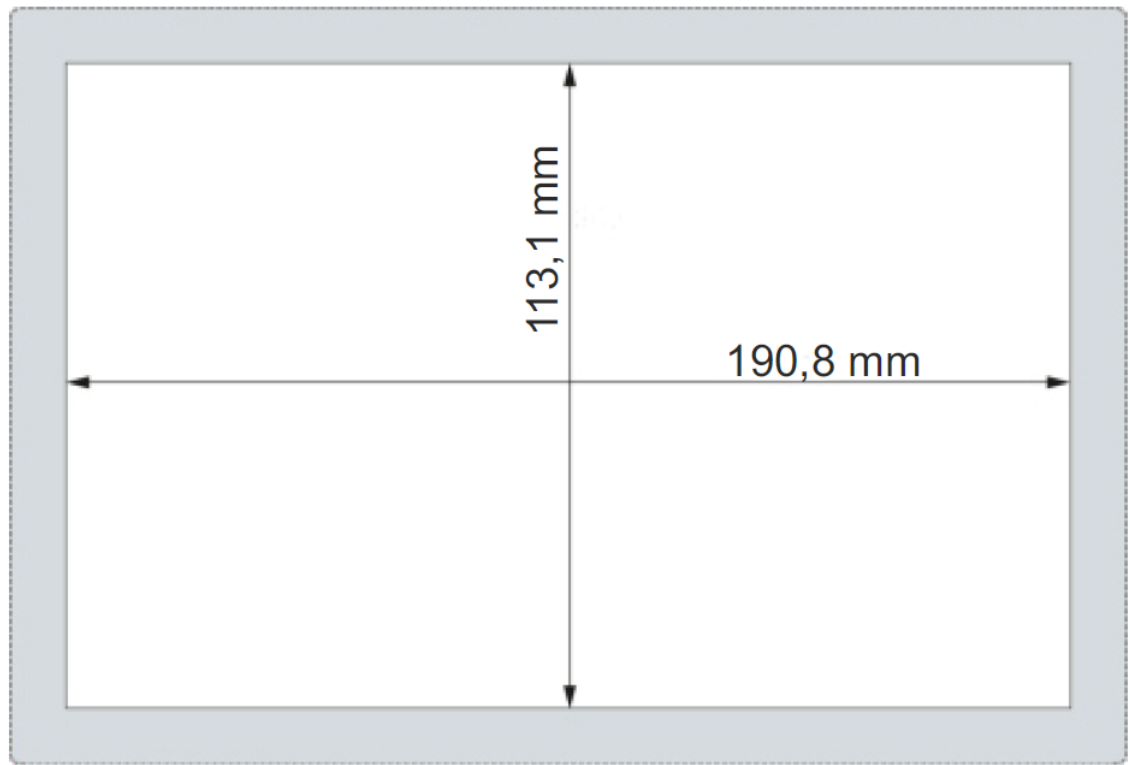
Abb. 10: Montageausschnitt DC-Rack 7
