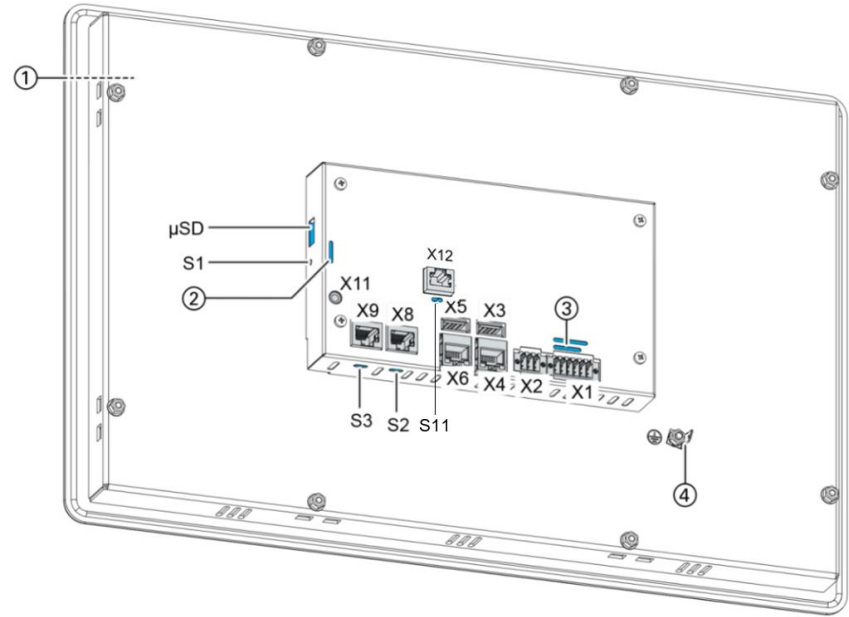
Abb. 4: Übersicht DC-Pro 10/15 (Rückseite)
