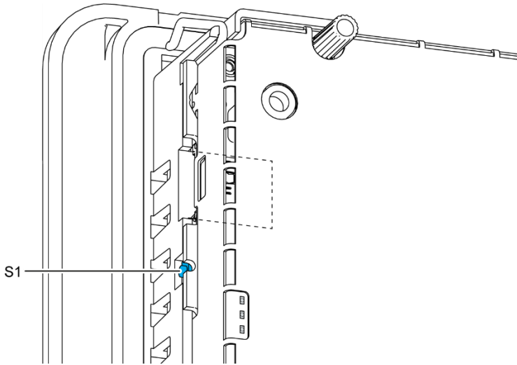
Abb. 52: Funktionstaster (S1)
