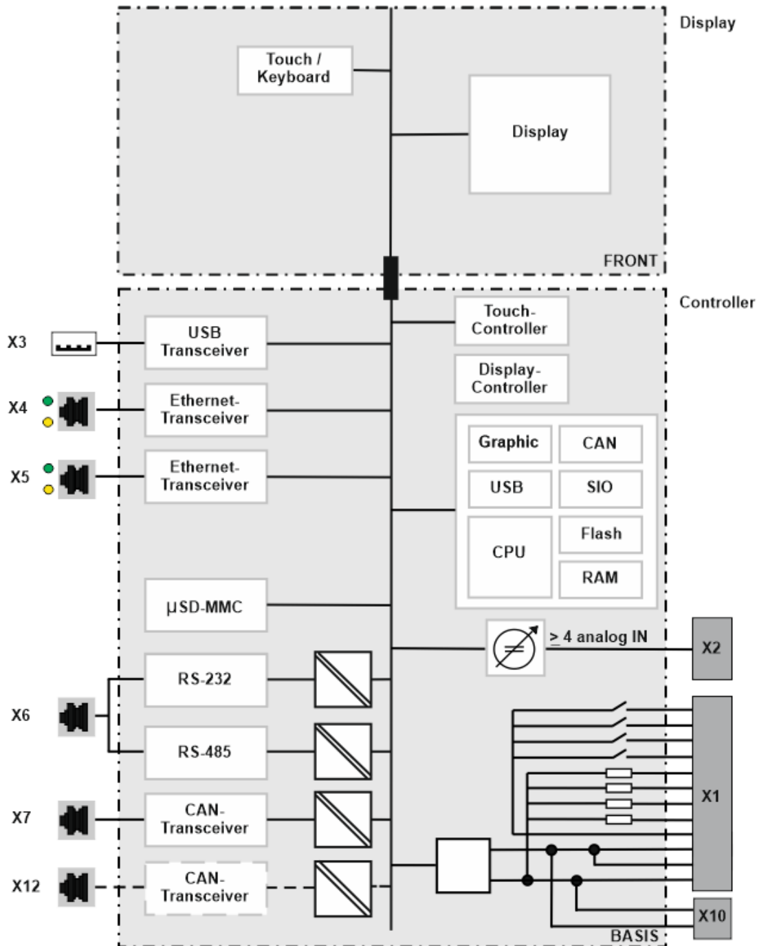
Abb. 28: Blockschaltbild DC-Pro
