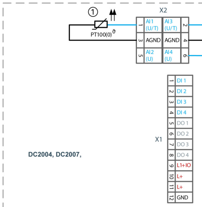
Abb. 38: Anschlussbeispiel: Temperaturmessung
