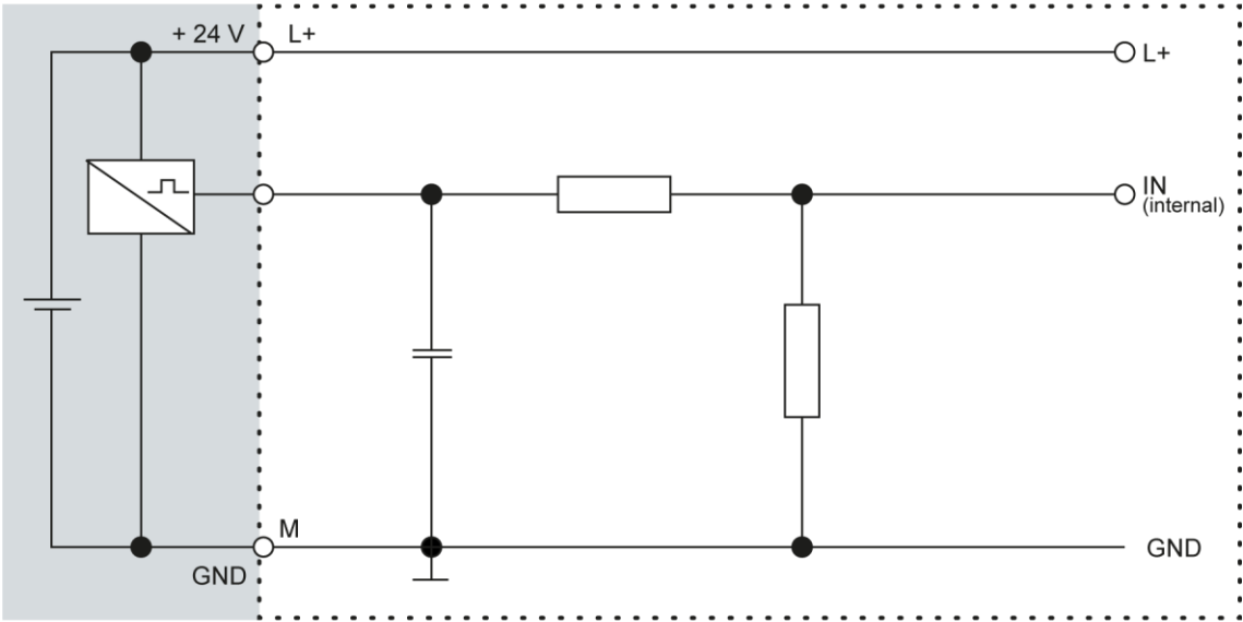
Abb. 32: Prinzip-Schaltbild Eingang, plusschaltend
