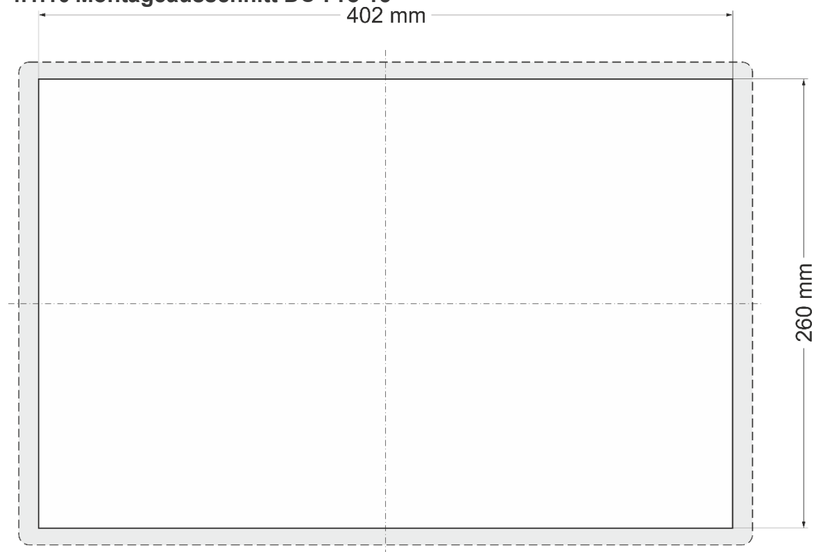
Abb. 14: Montageausschnitt DC-Pro 15
