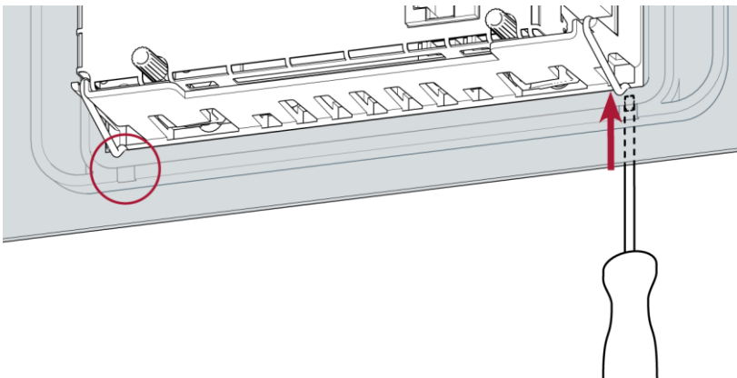
Abb. 53: Spannkammern lösen (DC-Pro 4/7)
