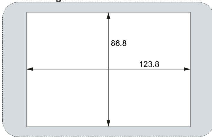
Abb. 6: Montageausschnitt DC-Pro 4
