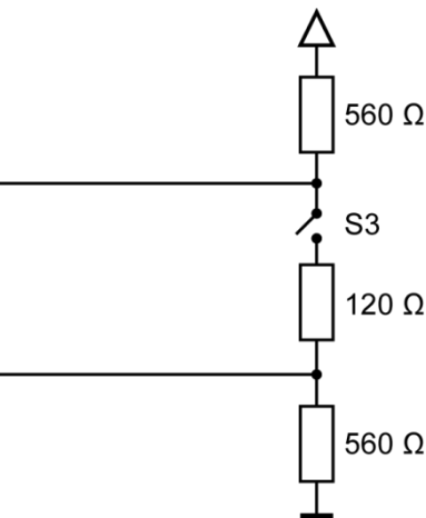
Abb. 44: RS-485 zuschaltbarer Abschlusswiderstand
