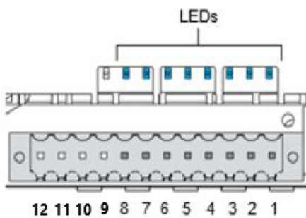
Abb. 25: DC-Pro 4/7 und DC-Rack 7 Spannungsversorgung Stecker X1 mit Power-LED
