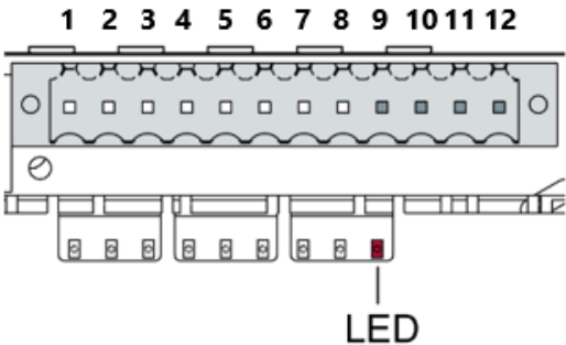
Abb. 29: Digitale Ein- und Ausgänge DC-Pro Stecker X1 mit LEDs 1 bis 8, einreihig
