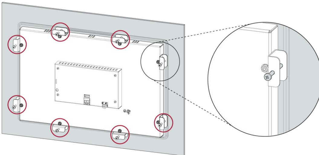
Abb. 24: Spannklemmen festschrauben
