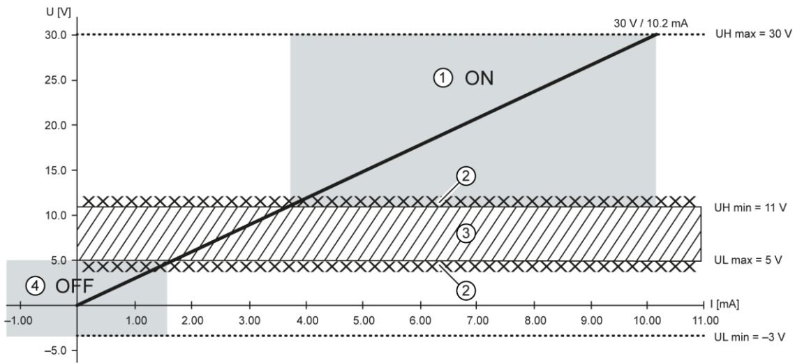
Abb. 33: Betriebsbereiche der digitalen Eingänge (Typ 1/3)
