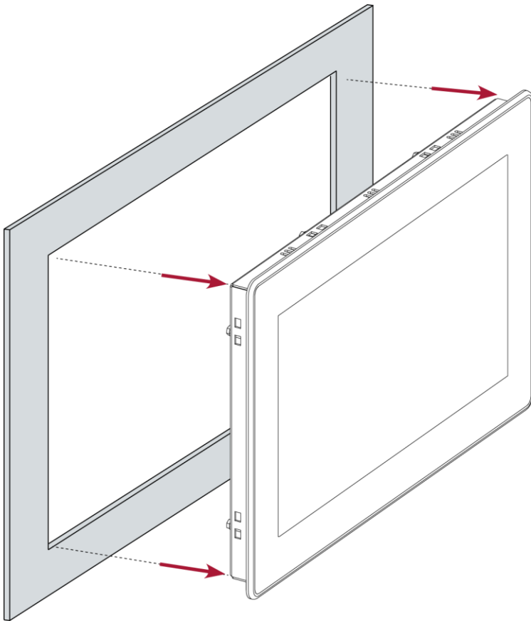
Abb. 58: Gerät aus Montageausschnitt schieben
