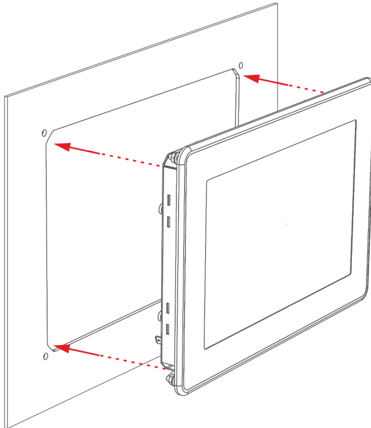
Abb. 19: Einsetzen in Montageausschnitt
