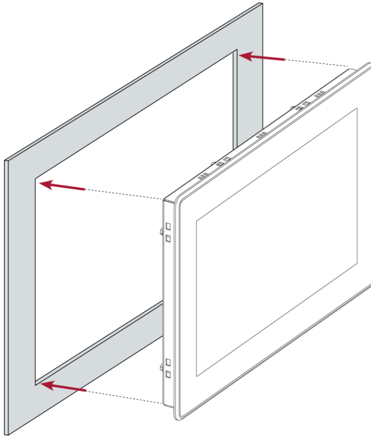
Abb. 22: Einsetzen in Montageausschnitt
