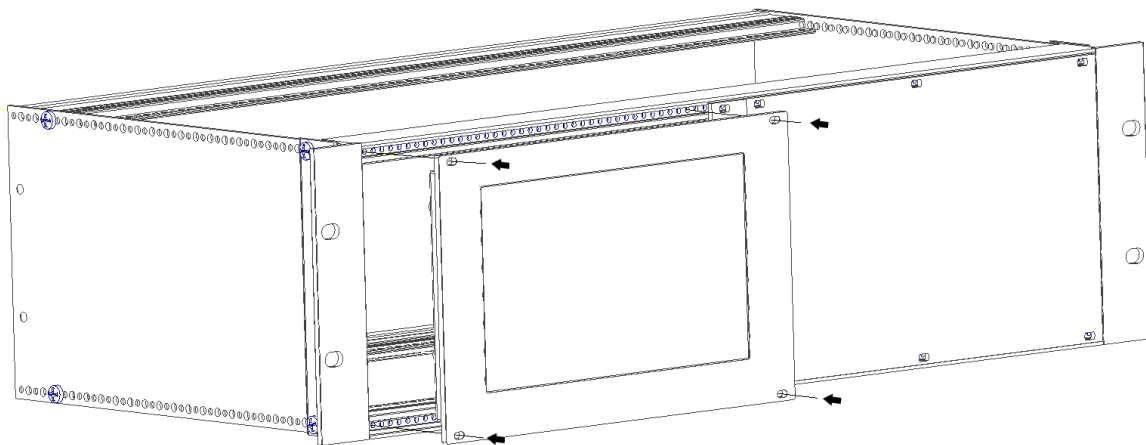
Abb. 18: Gerät in Montagerahmen 3HE einlegen und mit 4 Schrauben befestigen
