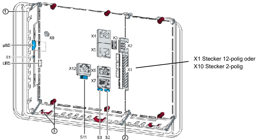
Abb. 1: Übersicht DC-Pro 4 (Rückseite)
