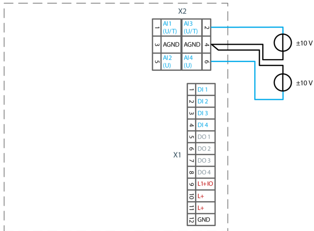
Abb. 37: Anschlussbeispiel: Spannungseingang
