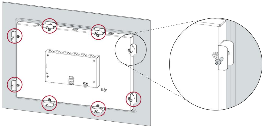
Abb. 56: Schrauben lösen
