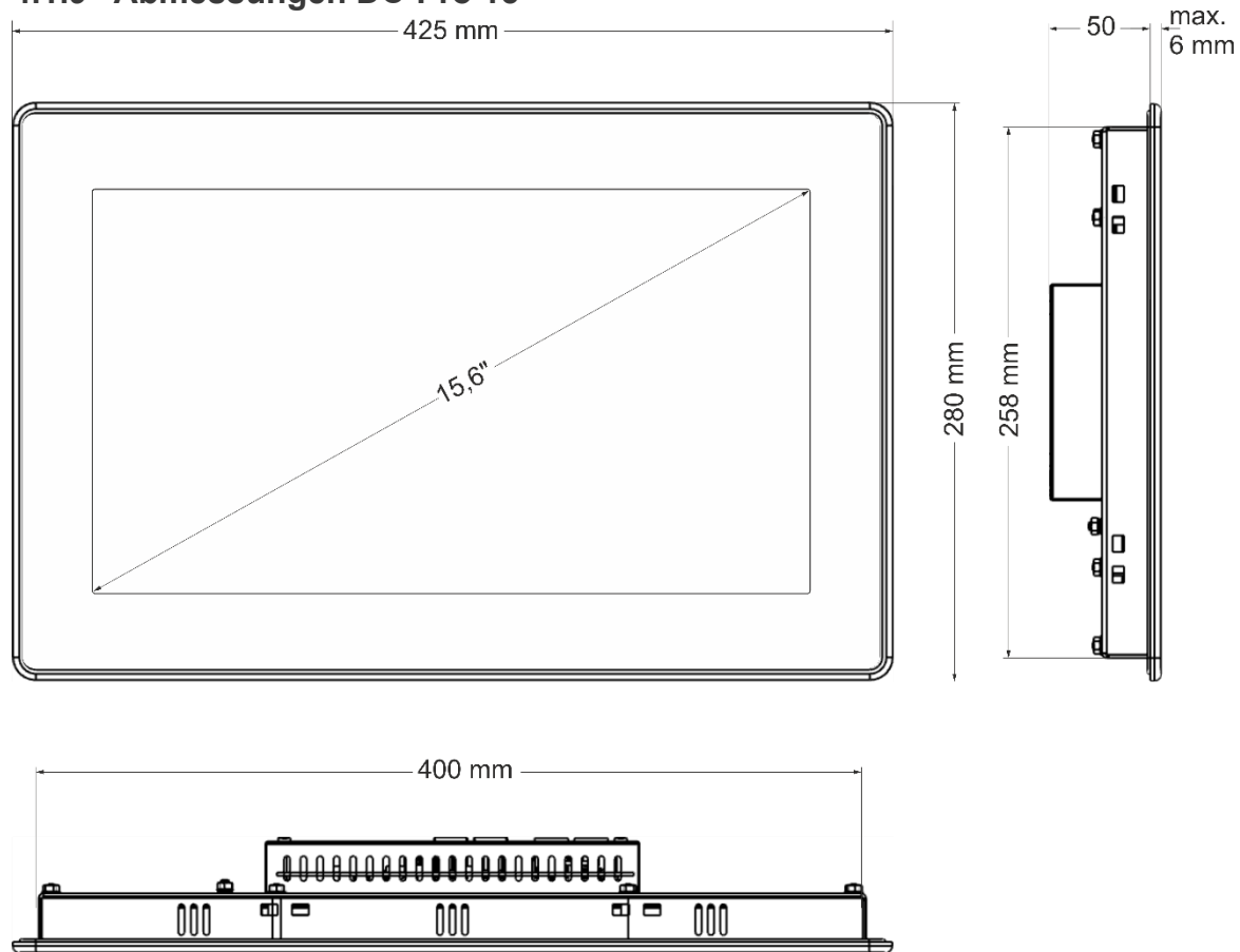
Abb. 13: Abmessungen DC-Pro 15
