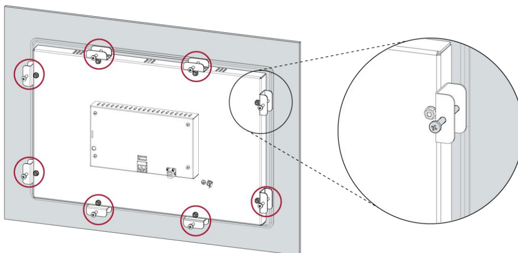
Abb. 21: Spannkammern festschrauben
