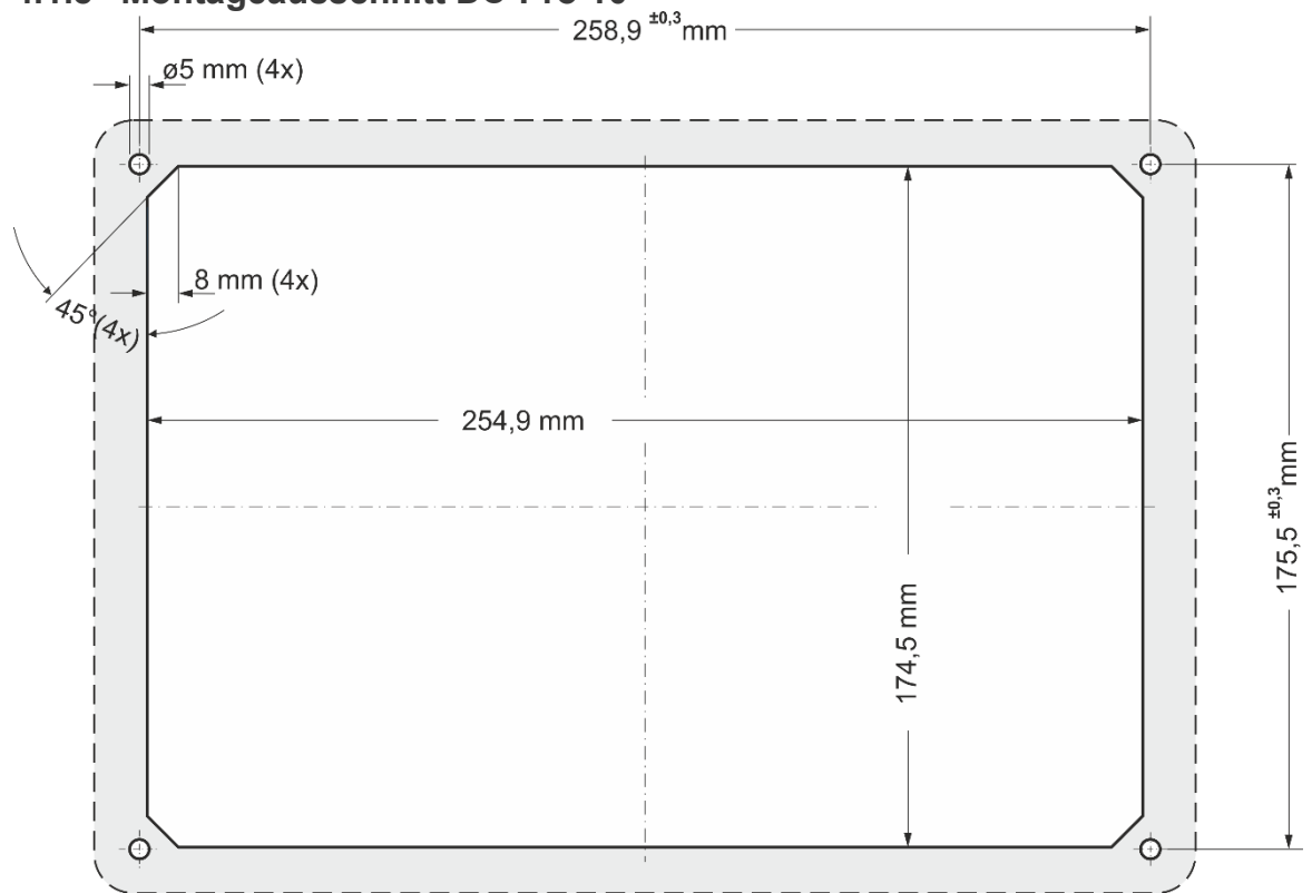
Abb. 12: Montageausschnitt DC-Pro 10
