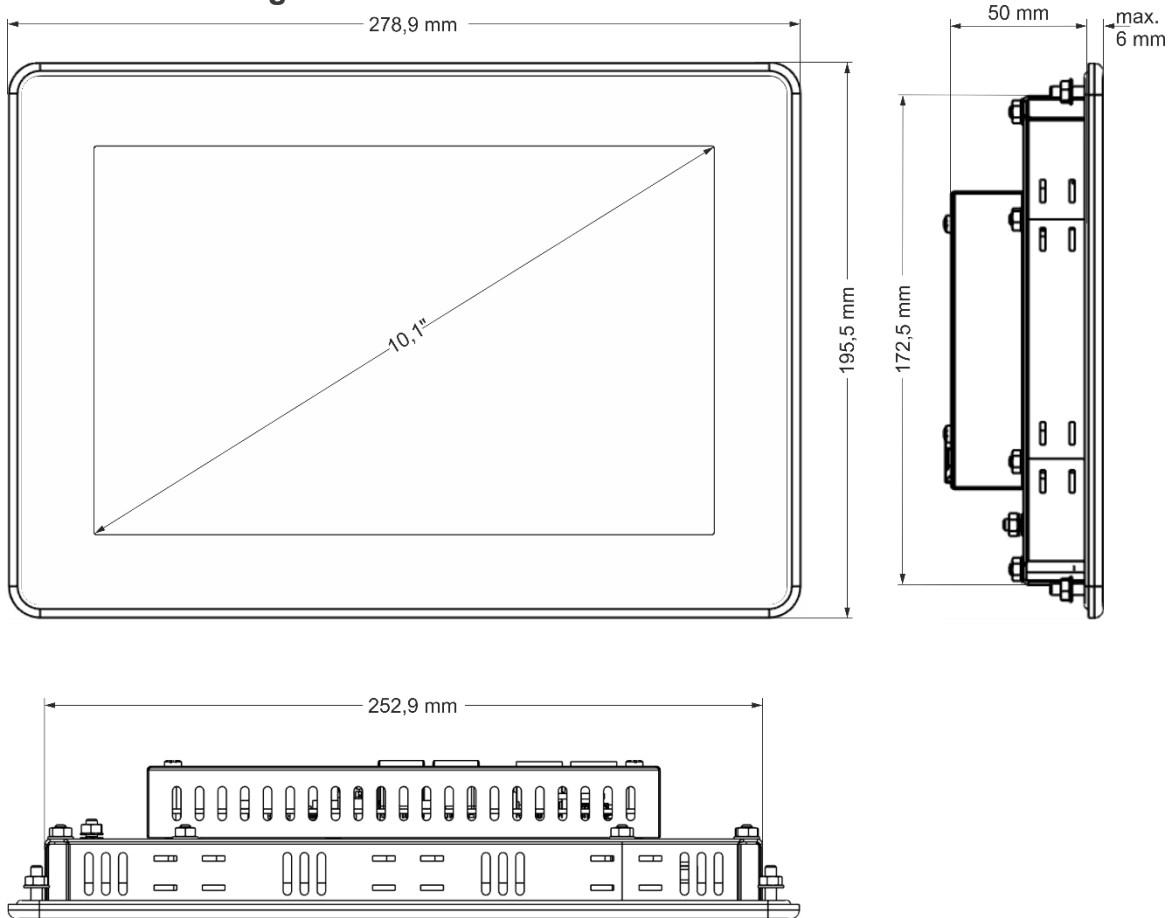
Abb. 11: Abmessungen DC-Pro 10
