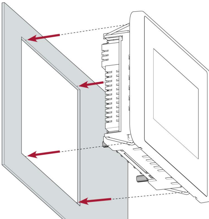
Abb. 16: Einbau in Montageausschnitt, Beispiel mit 4 Befestigungsklammern
