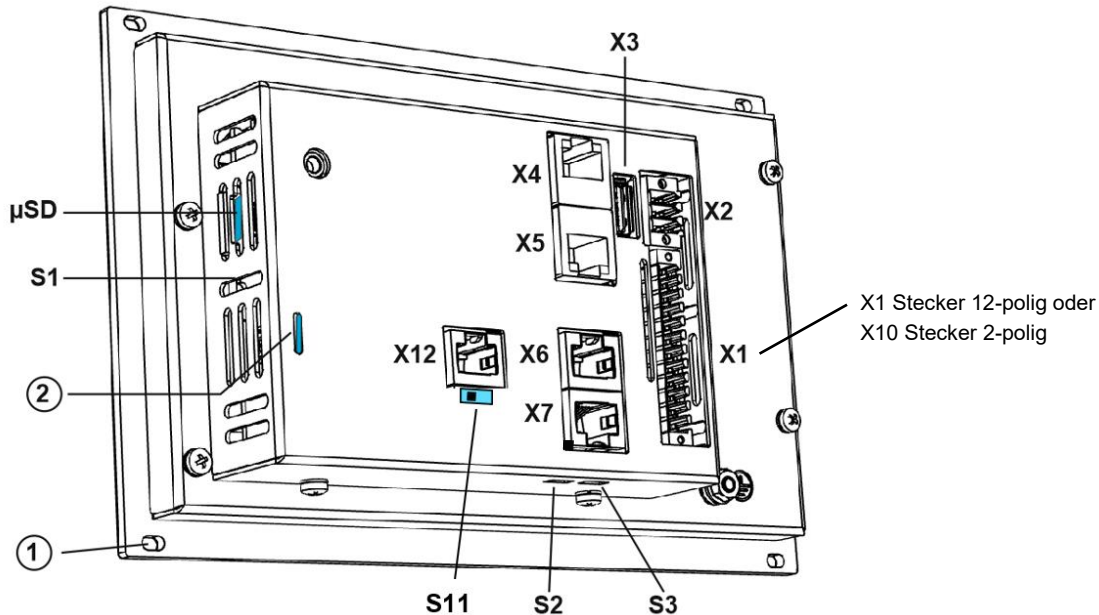
Abb. 3: Übersicht DC-Rack 7 (Rückseite)
