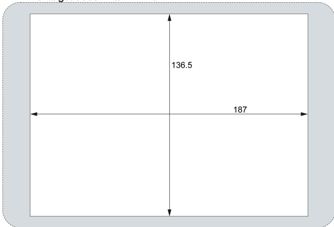
Abb. 8: Montageausschnitt DC-Pro 7
