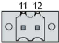
Abb. 26: DC-Pro 4// und DC-Rack 7 Spannungsversorgung Stecker X10
