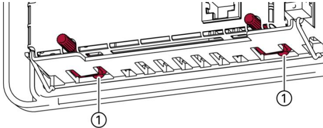
Abb. 15: Drehriegel offen
