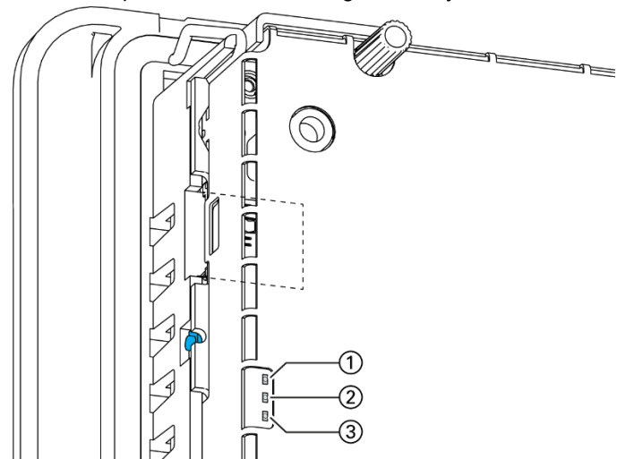
Abb. 51: Positionen der Betriebsstatus-LEDs
