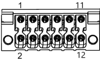
Fig. 19 : Analogue inputs (U/I/PT) X12
