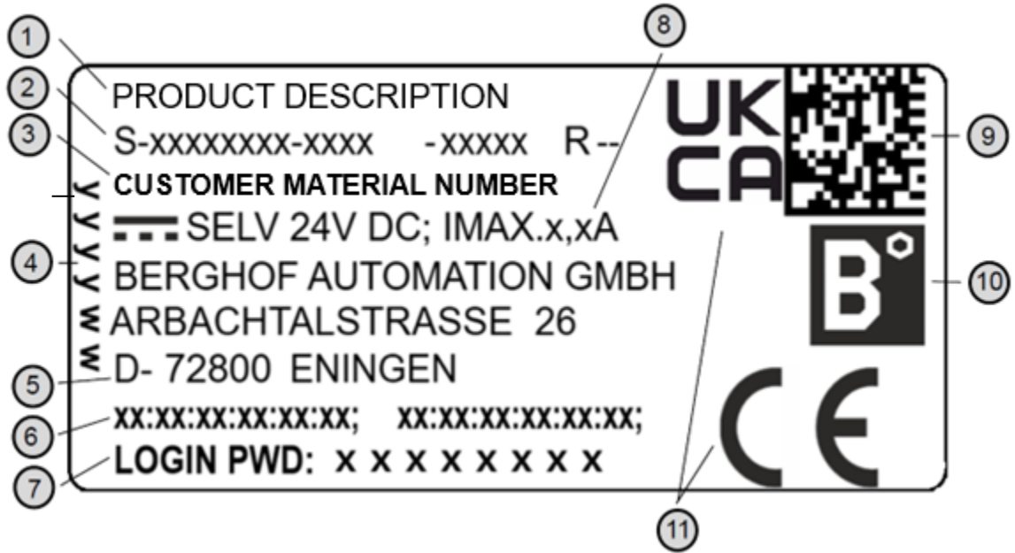
Fig. 37: Type plate
