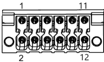
Fig. 19 : Analog inputs (U/I/PT) X12
